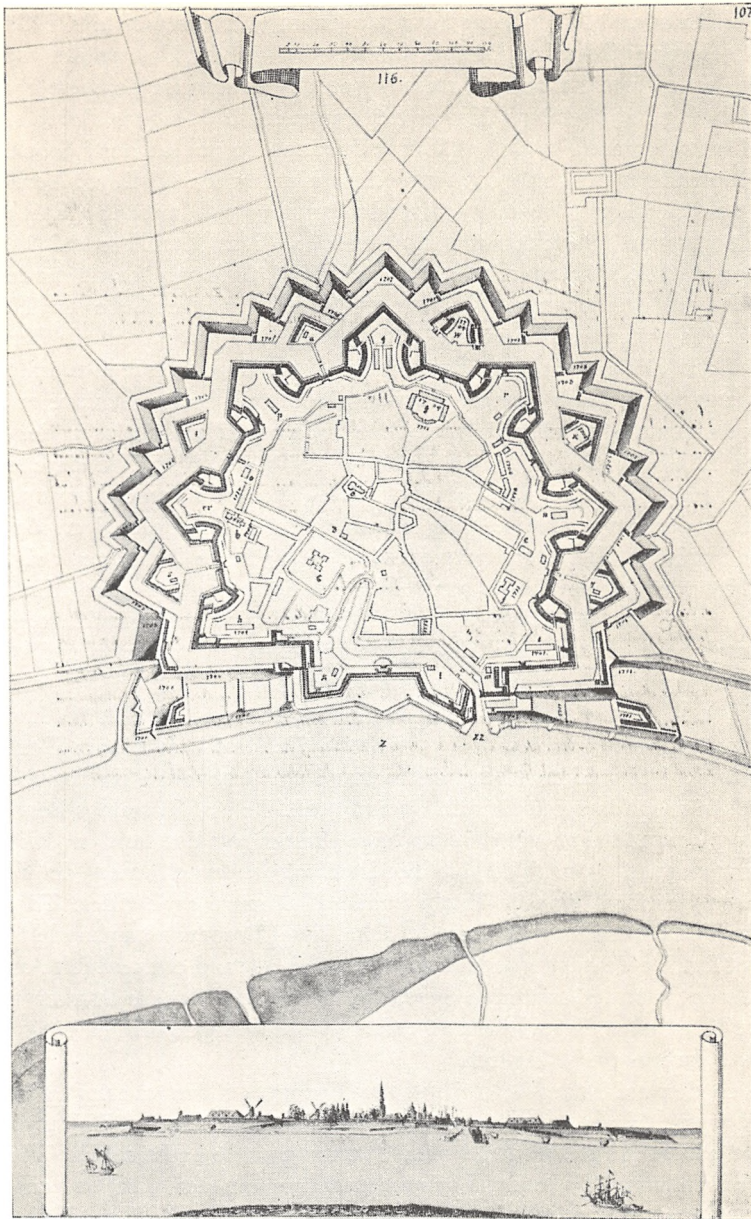
Fig. 75. Fæstningen Tønning ca. 1700. Tegning i Zacharias Wolf: Practische Kriegsbaukunst nach vieljähriger Selbsterfahrung. Det kgl. Bibl. fot.
