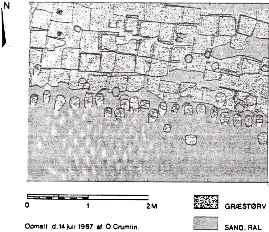
Plan af vestenden af centrale pælerække
