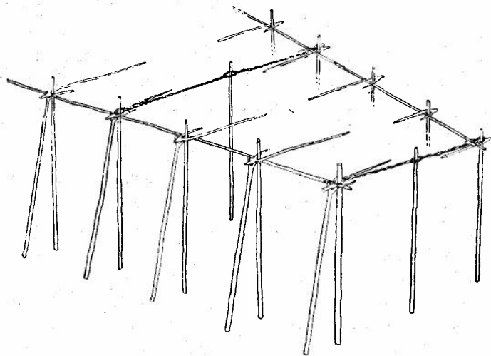
Fig. 5. Skema for fagkonstruktionen for den i fig. 4 viste træbygning. Eft. Dyggve.
