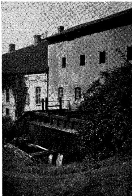
Fig. 13. Gudse Vandmølle (Nr. 44). S. B. fot.
