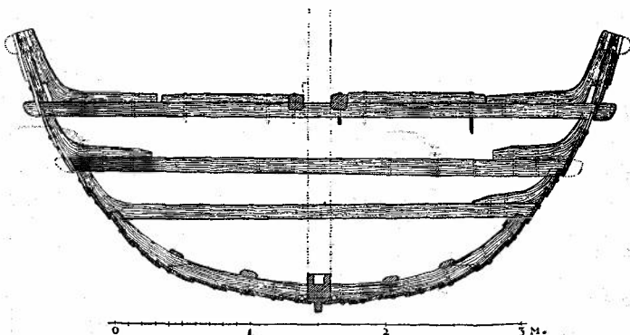
Fig. 7. Tværsnit af Kalmarskibet fra o. 1250 tegnet af H. Åkerlund.
