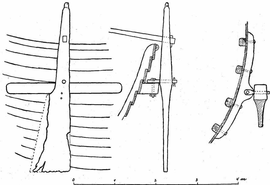
Fig. 4. Rorets ophængning.
