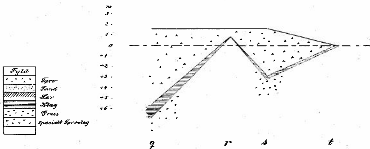
Profiler, tegnede af Landinspektør Axel Johansen efter Borejournaler.
