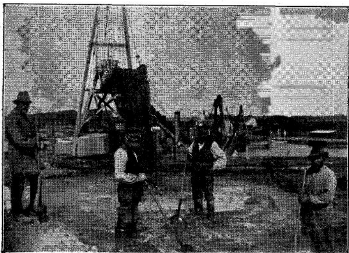
Opmudret Fyld udsprøjtes.
