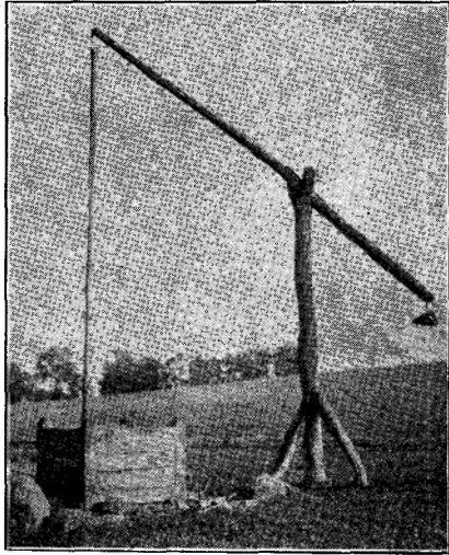
Fig. 4. Brøndvippe fra Stenstrup, Lyngesogn, Sorø Amt.
