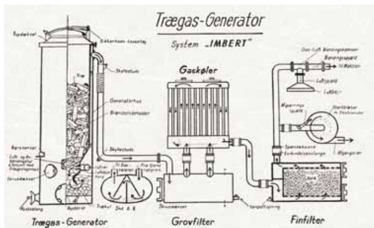
Skematisk fremstilling af elementerne i et gengasanlæg.
