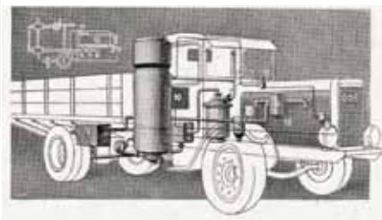
Skematisk fremstilling af elementerne i et gengasanlæg.
