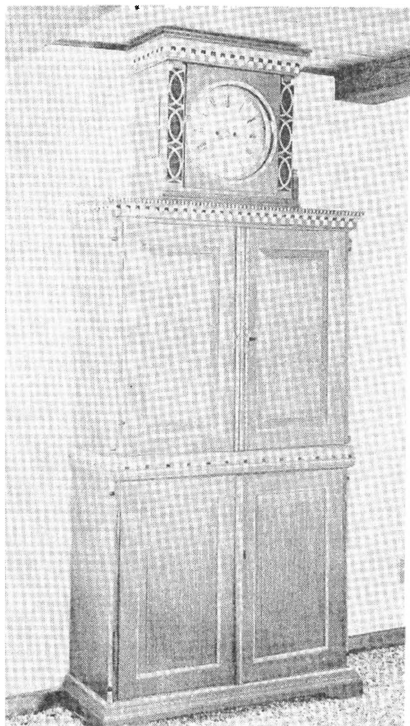
Lodur med pendul og slagværk indbygget i skab. Uret er signeret „Maabjerg 1833“. Det er fremstillet af Markus Sørensen, Maabjerg. Skabet, det er bygget ind i, måler i højden 197 cm og i bredden 80 cm. Privat eje på gård i Gettrup, Thy.
