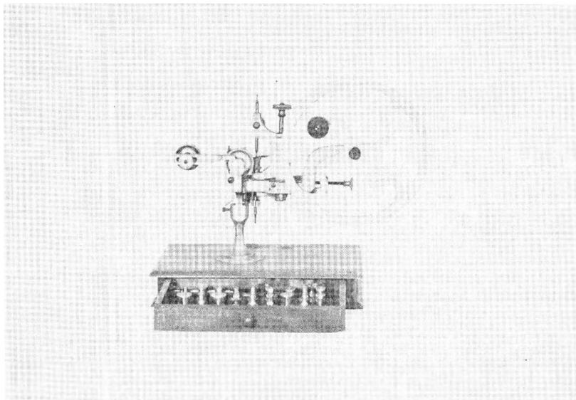
Fræsemaskine beregnet til fremstilling af tandhjul. Dette hånddrevne eksemplar har sidst været anvendt i Vestervig i Tby. Maskinens mål er 32 x 27 cm.
