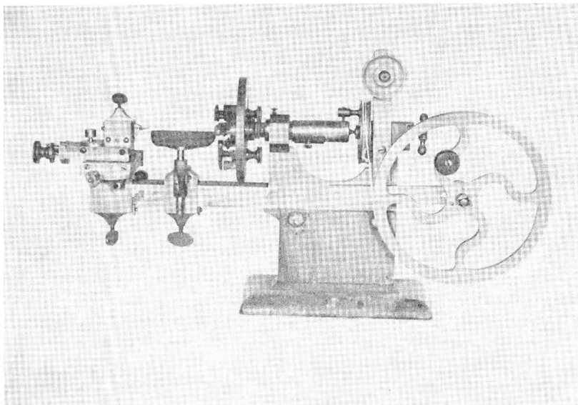
Plandrejebænk brugt af urmagere til fremstilling af bl. a. talkrans til standure og lågkapsler til lommeure. Sidst anvendt i Vestervig i Thy. Maskinens mål er 61 x 31 cm.
