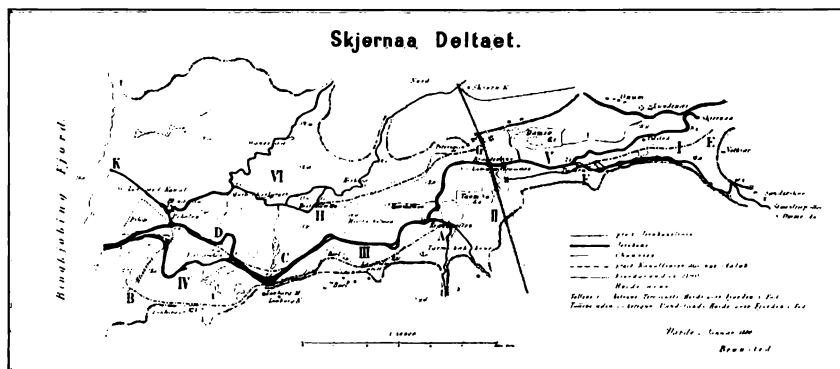
Skjernå-deltaet, som ingeniør Brønsted udformede det i 1880, tre år inden han og landinspektør Lauridsen udarbejdede deres forslag til Skjernå-kommissionen. Ill.: Det Danske Hedeselskab.
