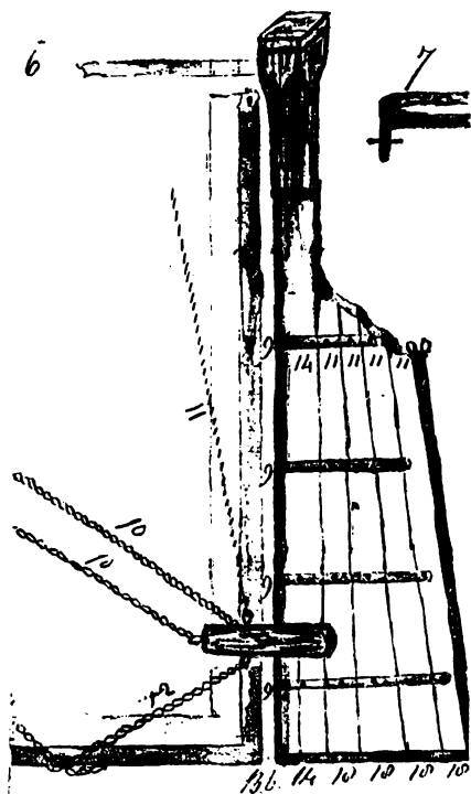
Kommandør Paters skitse til det Pakenham rør, der blev lavet til St. George ombord på Cressy: 6. rorpinde, 7. tømmerkonstruktion, der skal holde den øverste del af roret fast til dækket, 9. afstivninger, 10., 11. og 12. kæder, der fastholder roret, 14. topstang, der udgør rorstammen og bag denne er der boltet rundbolter (mærket II), 18. jernvægt.
