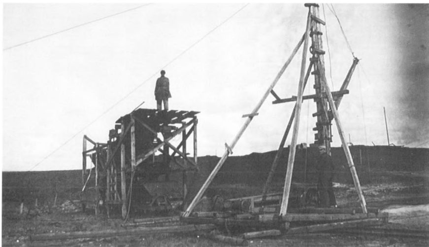
Spil med svingbom, der trækker kulsplandene op til manden på stilladset. Motiv fra Fiscbers leje i Nørre Viium. (Foto: Privat)
