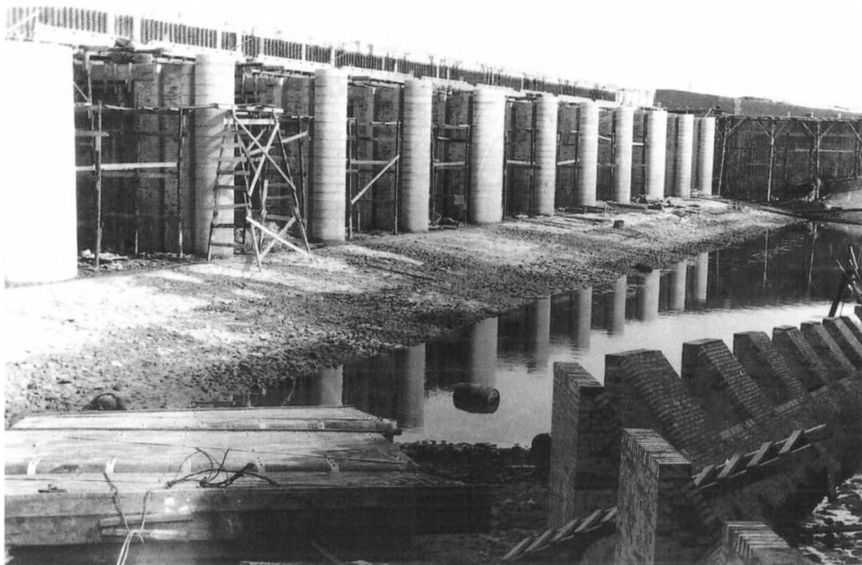
Tør sluse fra vest. Manøvre gangsmuren over slusekamrene er opmuret. Forrest i billedet ligger 3 svære egetrasporte og venter på at blive løftet på hængslerne. Det tandformede murværk nærmest t.h. er strømbrydere, der skal nedsætte vandets hastighed ved slusens bund for at forhindre underskæring. (A. Grimstrup)
