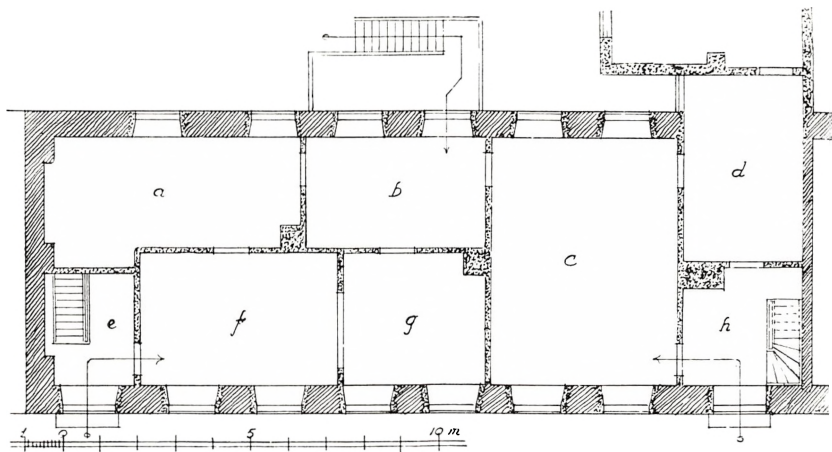
Fig. 2. Grundplan over første Stokværk af gl. Matr. Nr. 210, St. Peders Kirkeplads 12), hvor Chr. Bonnesen havde Restauration 1848—54. a, b, e, f og g svarer til Restaurationslokalerne med Entré og Læsestue. c maa være „Salen“. Opmaalt og tegnet af Arkitekt J. Tidemand-Dal, Næstved, 1958.
