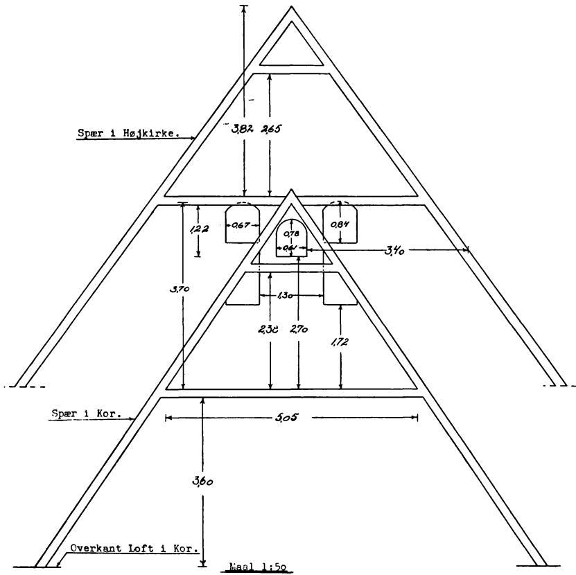
Korets og Højkirkens Tømmerværk med Glanhullerne. Opmaalt og tegnet af Børge O. Andersen.
