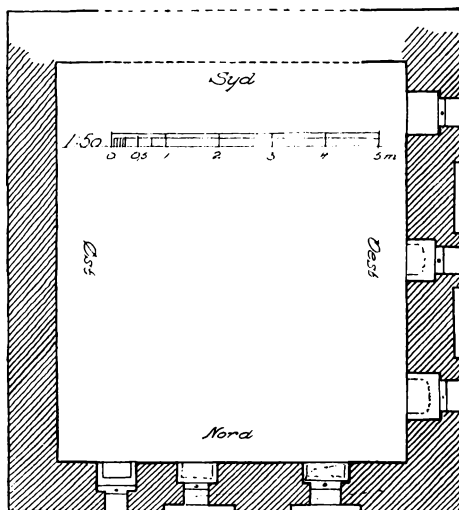
Skydeskaar i Taarnets andet Stokværk, opmaalt og tegnet af S. A. Claudi Hansen.
