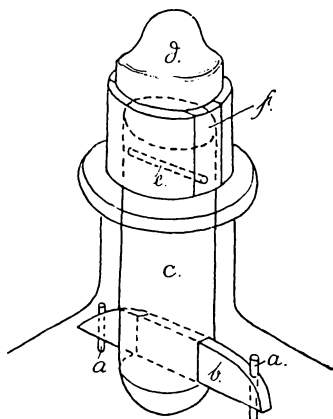
Arkitekt H. Zangenberg: Told til en Flaske med Rok eller Garnvinde (Haspe), a) Tværpinde i Splitten, b) Splitten, c) Tolden, d) Hovedet til Tolden, e) Tværpind, der holder Told og Hoved sammen, f) små Skodder, der dækker Tværpindens Ender.
