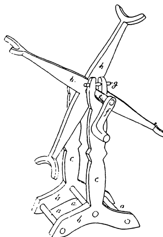
Arkitekt H. Zangenberg: Garnvinde (Haspe) til at sætte i en Flaske, a) Tværpinde, b) Fodstykker, c) Opstandere, e) Aksel, f) Haandstag og Sving, g) Pind over Akselen, h) Vingerne.
