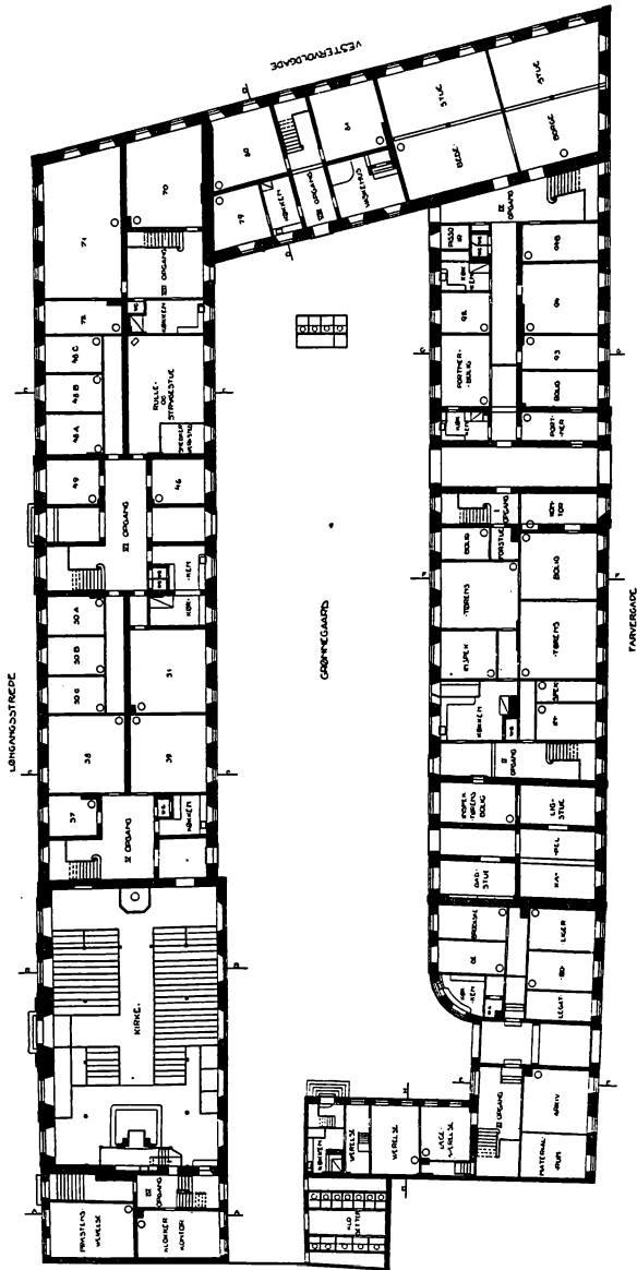
Fig. 2. Plan af Vartovs Stueetage, 1915.
