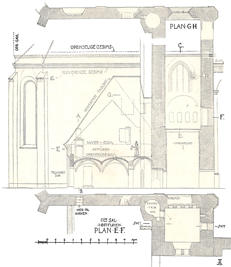
Fig. 2. Korets Nordside, med Snit gennem Sakristi og Taarn. Plan E—F, fornedet, viser Korets Nordmur i Højde med Sakristiets Tagfod og Taarnets næstnederste Stokværk. Plan G—H, foroven, Kor-muren noget under Kirkens Gesimshøjde.
