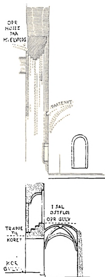
SNIT C.D. ØVERST. - A.B. UNDERST
