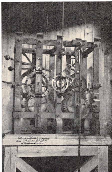
Sølvgades Skoles gamle Smedejernsurværk, der nu fungerer i Ryslinge Kirke paa Fyn. Opsat dér 1899. Fot. 1947.
