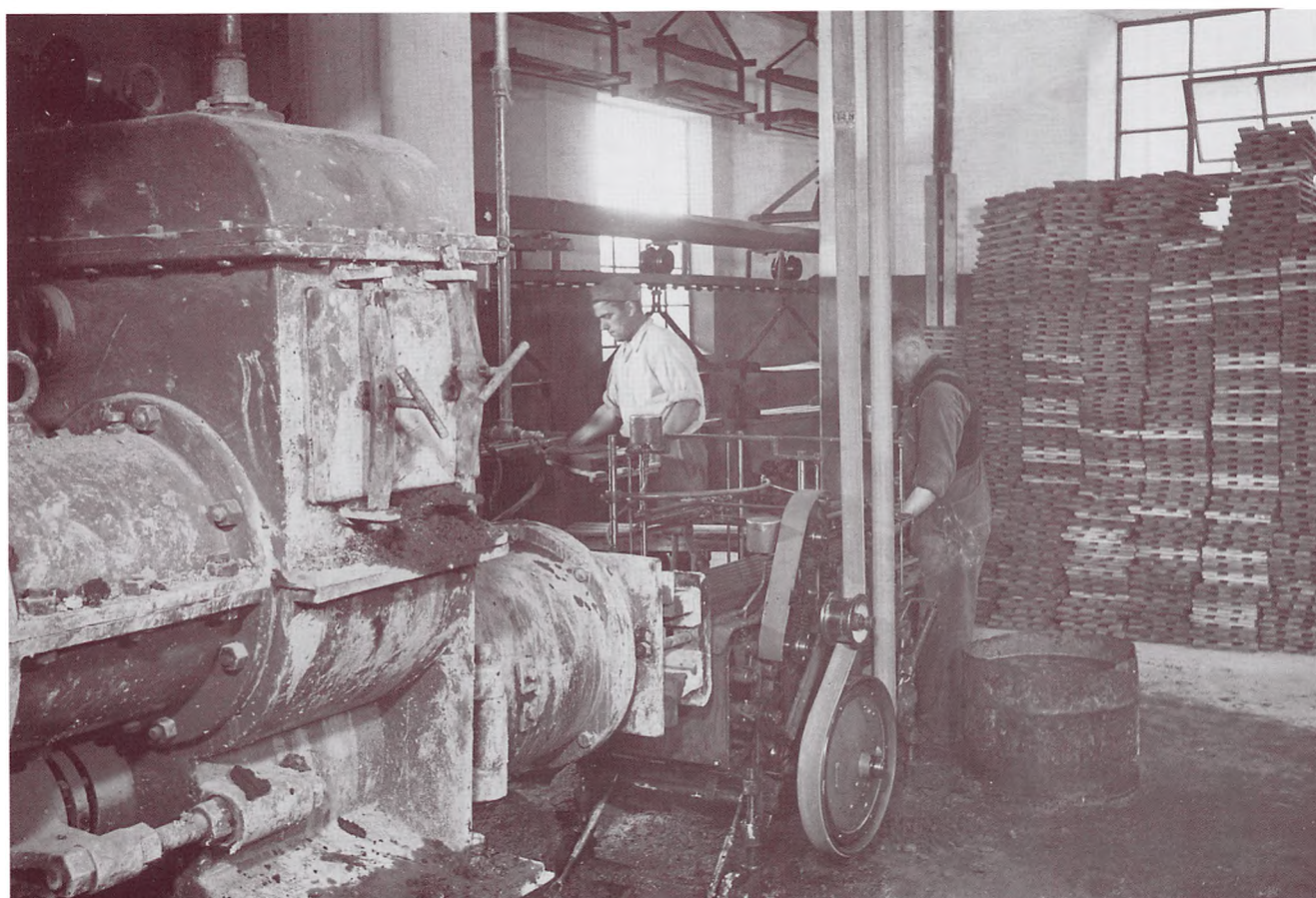
Strygemaskine, Søndre Værk, Skarrehage Molerværk, ca. 1953.
