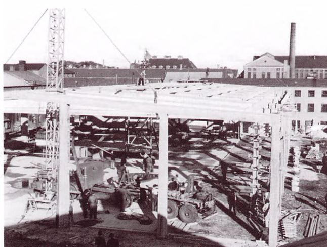
Den ny støbehal opføres i 195x. Byggeriet var det første af sin art i denne del af landet. De store bjælker blev leveret af Jydsk Betonelementfabrik ved Kolding, entreprenør var firmaet Ejner Mikkelsen A/S, Aarhus.
