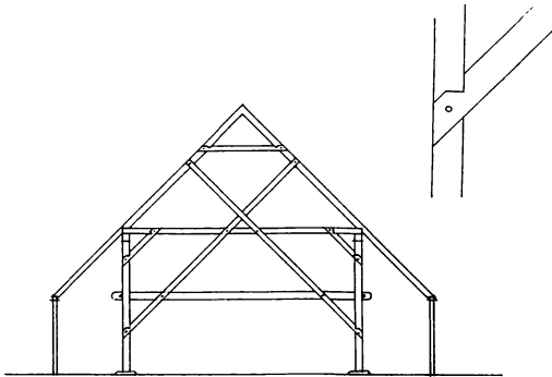
Fig. 9. Tværsnit af Laden visende Tømmerkonstruktionen. Paa Højde med Nederbjælken gik en vandrer Stiver fra Benet ud til Murremmen, ikke vist paa Figuren.
