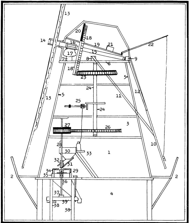
Skematisk tegning af mølle
