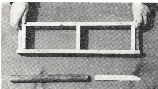
Fig. 4. Strygeform, Stok til Afglatning og Trækniiv. Stokken blev rullet hen over de færdigstrøgne Sten, dernæst tog Strygeren fat i Formen paa den her viste Maade og bar Stenene ud paa Strygepladsen
