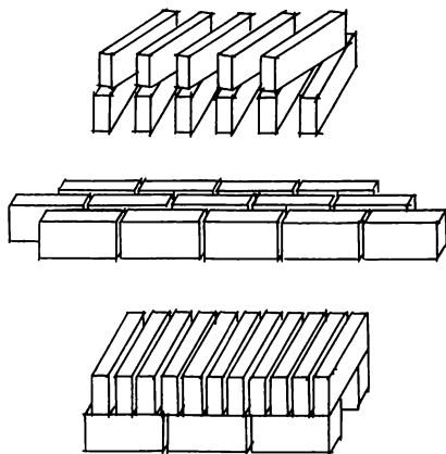
Fig. 5. Øverst Rankerne i de nederste 13 Lag i Ovn, denne blev fyldt fra »Bunden« af, Rankerne gik fra Side til Side.
