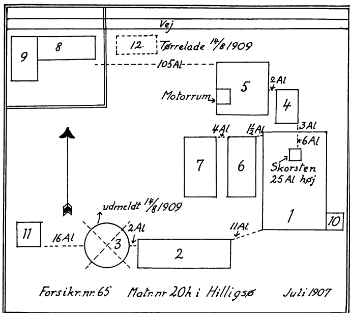
Fig. 2. Grundplan over Teglværksbygningerne efter Skitse fra 1907, bør sammenholdes med Kortet Fig. 1. Tørreladen Nr. 12, Bygningerne Nr. 5 og 4, den lille Tilbygning Nr. 10 samt Skorstenen paa Nr. 1 er kommet til efter 1906. Nr. 1 er Højovnen, Nr. 2 den store Tørrelade, Nr. 6 og 7 de smaa Tørrelader, Nr. 3 Æltemaskinhuset, Nr. 11 Baadehuset, Nr. 8 og 9 Beboelseshus og Stald. Strygepladsen laa mellem disse Bygninger og Vejen, de to »Traj« laa lige Nord for Æltemaskinhuset, ved Baadehuset var der et Spil til Ophaling af Baadene. I Juli 1875 var Nr. 1, Nr. 2, Nr. 3, et Beboelseshus og en Tørrelade færdige, de to sidste er muligvis identiske med Nr. 8 og Nr. 6
