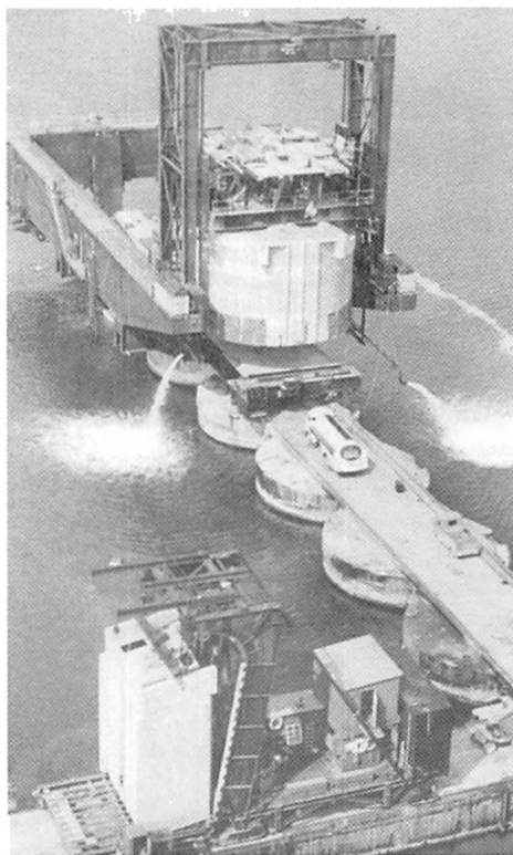
Den specialbyggede skotske kran, der satte betonkasserne på plads på havbunden. Kranen vejede 600 tons. Foto: Chr. Schröder.
