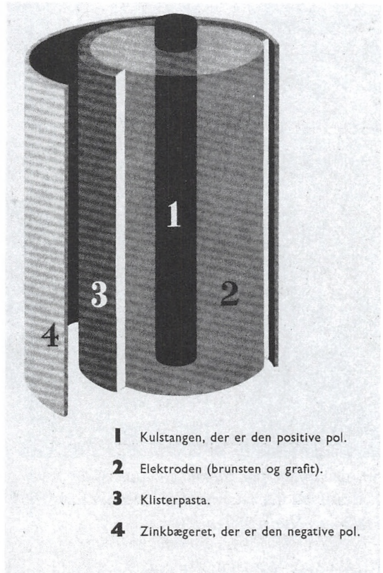
Snit af et brunstensbatteri.
