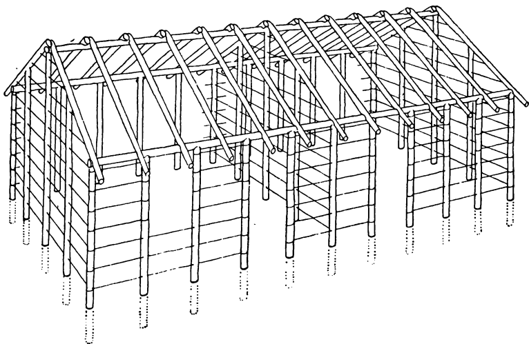
Træ- og Staaltraadsskelettet til et Barrohus.
