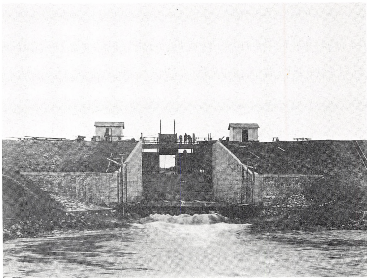
Frislusen. Billedet synes at stamme fra søens opfyldning i dec. 1920, hvor en del af åens vand ledtes gennem frislusen, hvorfor bundslusen ikke ses. Slusen ses bagfra, dvs. modsat søsiden. De øverste sluseportes funktionsmåde fremgår tydeligt.
