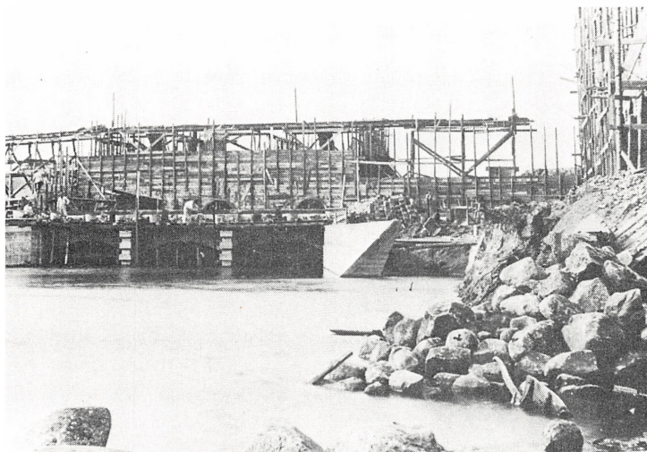
Fig. 26. Kraftstationen under opførelse. Billedet tilhører Lokalhistorisk Arkiv i Bjerringbro. Ukendt fotograf.
