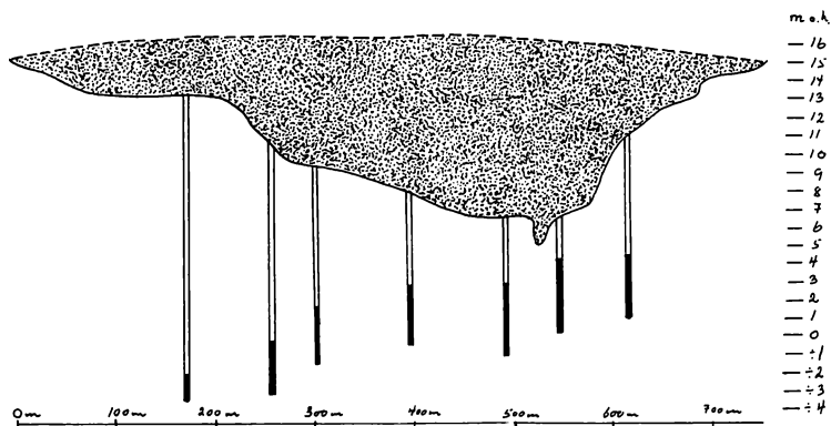
Fig. 23. Tværsnit af Gudenådalen på hoveddæmningens plads. Højden stærkt overdrevet i forhold til længden. Fuldt optrukken linie angiver oprindelig overflade - den punkterede overfladen af dæmningen. 7 borehuller angivet - sort betegner glimmerler. Det ses, at man til venstre måtte fjerne mere end 10 m overjord, før leret nåedes. Efter hefte indeholdende planer til Gudenåcentralen uden titel og forfatterangivelse i Lokalhistorisk Arkiv i Bjerringbro.
