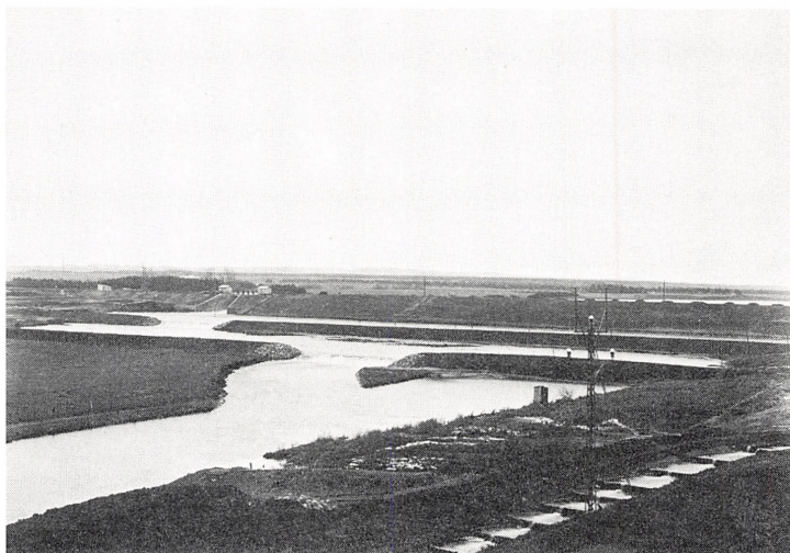
Fisketrappe, støttedæmninger og hoveddæmning set fra kraftstationen - søen skimtes bagved hoveddæmningen. Billedet er sikkert taget samme dag som det foregående og altså under søens opfyldning, hvor en del af åens vand fik lov at løbe gennem frislusen. Ved sikringsdæmningen ses det passere styrtene, hvorved der opstår små vandfald. Det lille hus i midten var »et lille hus« til brug for arbejderne. Masten er den første på højspændingsledningen til Århus.
