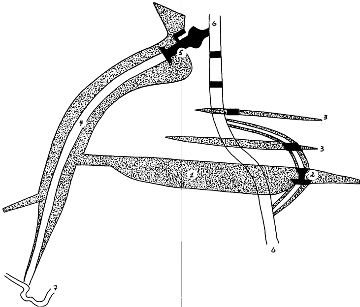
Fig. 22. Anlægsplan. Forklaring: 1) Hoveddæmning. 2) Frisluse. 3) Støttedæmninger. 4) Tilledningskanal. 5) Kraftstation. 6) Gudenå. 7) Tange å. Efter hefte indeholdende planer til Gudenåcentralen uden titel og forfatterangivelse i Lokalhistorisk Arkiv i Bjerringbro.
