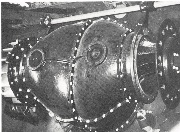
Fig. 20. Dobbeltturbine. Venstre halvdel intakt - højre åben så selve turbinen med de buede skovle ses. Fotograf: Jørgen Hedelund. Billedet tilhører Tage Kirkegaard, Tange.
