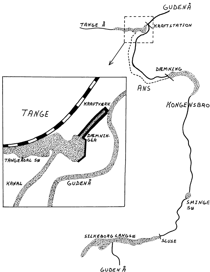
Fig. 18. Skitse af Fabers og Thomsens plan. Stiplet linie: kanal. Bearbejdet efter S. A. Faber og Kr. Thomsen: Forslag til Kanal- og Kraftanlæg ved Gudenå, 1910, fig. 1. Udsnittet viser de forhold, der ved planens gennemførelse ville opstå i Tange. Efter samme, planche X.
