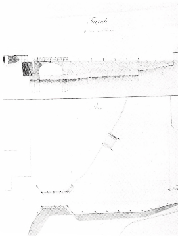
Fig. 2. »Tegning over Broe Arbeidet ved Colding, saaledes som samme er fuldført Aar 1808«. Facade af broen imod Fjorden.
