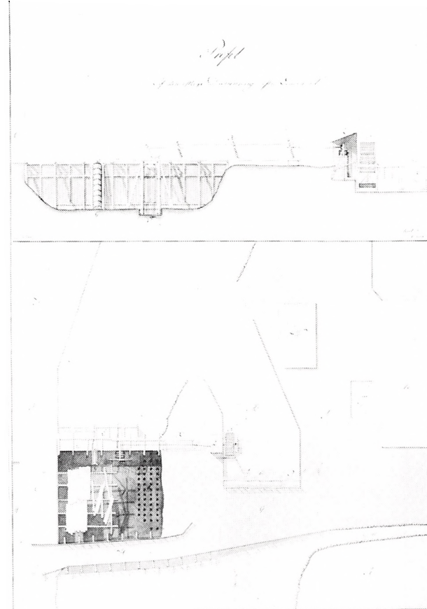
Fig. 4. Profil af den østlige dæmning.
