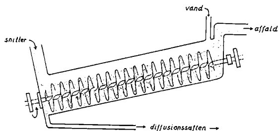
Skitse af diffusionsapparat
