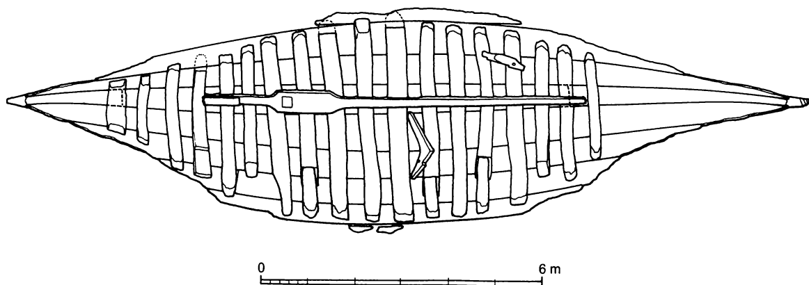
Plantegning af det udgravede vrag på bunden af Kolding Fjord udført af Fred Hocker, 2001.
