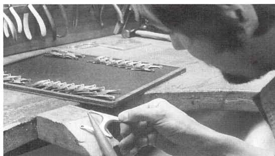
Øverst: På uvalsedde guldplader, ca. 2 mm tykke, aftegnes kædens enkelte led, hvorefter de savnes ud. Nederst: kædeleddet files, indtil den ønskede form er opnået.
