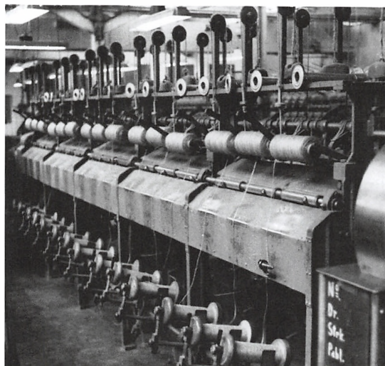
Det var et kompliceret maskineri, der skulle holdes gang i på Hørfabrikken. Foto ca. 1950.
