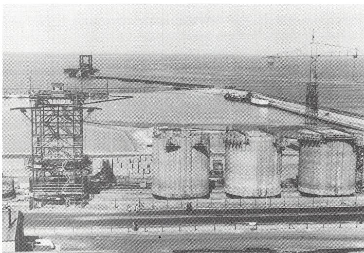
Den store skotske kran var nået ud på østre ydermole. I forgrunden tre af de kæmpemæssige beton-elementer. (Foto: Jens Steffensen).
