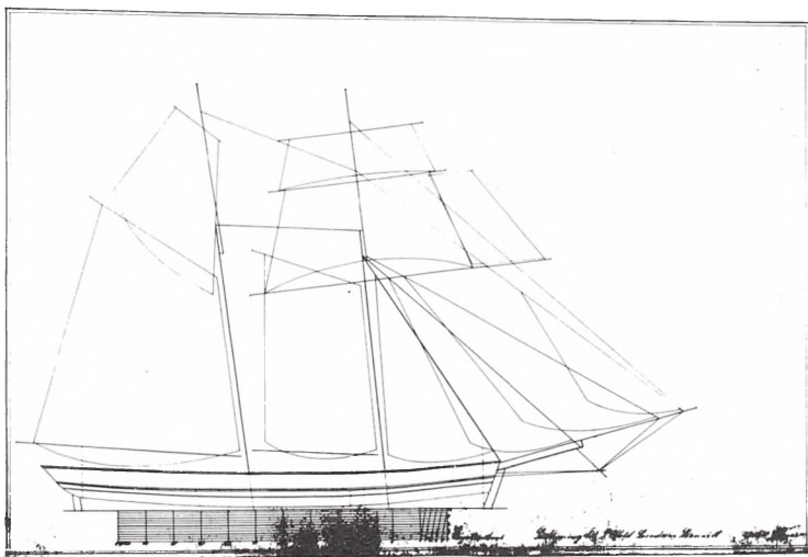
»Sejltægning til P. Kold Svendsens skonnert, Engelsk Maal« tegnet 19.12. 1861. Skonnerten er »Caroline og Sira«, der var bygget i Mandal i 1854 og forliste ved Søby i 1867. Mus. nr. THY 2304X34.
