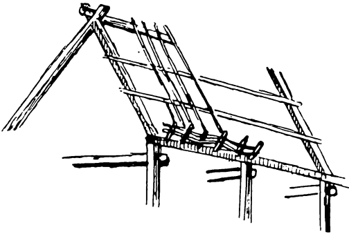
Fig. 3. Tagkonstruktion fra Rebild, Høllum h., Aalborg amt (Skitse af R. Mejborg). Spærene staar paa tagremmen og krydser hinanden foroven. I krydset foroven ligger rygaasen. Parallelt med rygaasen nede paa spærenes sider er anbragt to sideaase. I tagremmen er boret nagler og mellem disse er der flettede grene. Fra tagremmen op over sideaasene til rygaasen ligger der rafter (paa skitsen er der kun vist fire). Oven paa rafterne har der ligget fasttrampet lyng.
