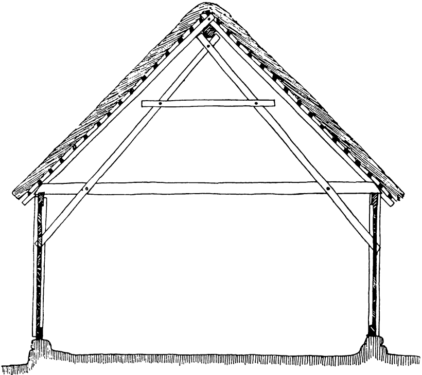
Fig. 7. Tværsnit gennem lade i Stannared, Himle h., Halland (efter M. Clemmensen, Bulhuse II).
