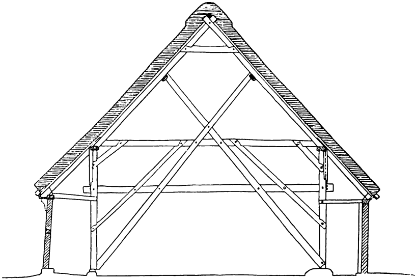
SNIT I LADE
