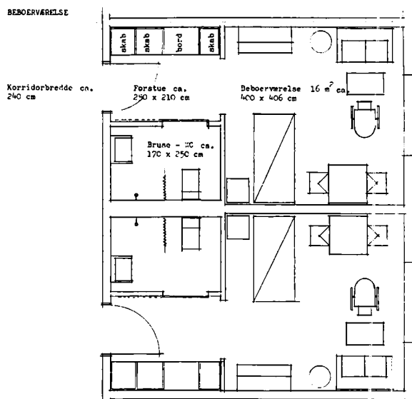
Tegning af 2 af de i alt 48 værelser for plejebeboere. Til hvert værelse hører der en forstue og et toilet- og badeværelse med bruse. Adgangen til værelser sker via en bred korridor. (Tegning af I/S Salling-Mortensens Tegnestue, Højbjerg).
