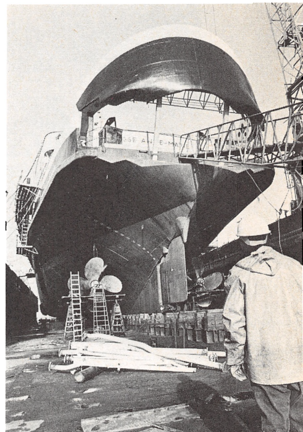
Hurtigfærgen Prinsesse Anne-Marie blev på Værtet savet igennem for at blive gjort ca. ½ meter højere. Det omfattende indgreb skabte plads til installering af et hængedæk til forøgelse af færgens personilskapacitet. Der blev brugt 69 håndbetjente donkrafte for at løfte færgens overbygning. (Foto: Ib Hansen)
