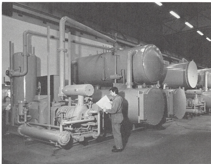
Disse store kølemaskiner, der er fremstillet af Thomas Ths. Sabroe & Co., blev i begyndelsen af 1974 sendt til Brasilien, hvor de skal benyttes ved bygningen af et dæmnings- og vandkraftprojekt. Maskinerne bruges til at nedsætte temperaturen på det støbemateriale, der anvendes ved bygningen. Herved opnår man at forlænge hærtningsprocessen, og det betyder, at betonen bliver stærkere. Værdien af anlægget er 3 mill. kr.; det er småpenge i forhold til den ordre, Sabroe fik i foråret 1974 på køle- og fryseanlæg til koreanske skibe. Ordren har en værdi af ca. 40 mill. kr. og er den største i firmaets historie.
