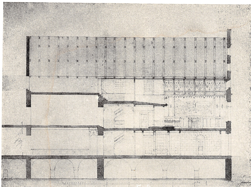
Fig. 8. Længdesnit gennem søndre Bygnings Forhus. Marts 1852.
