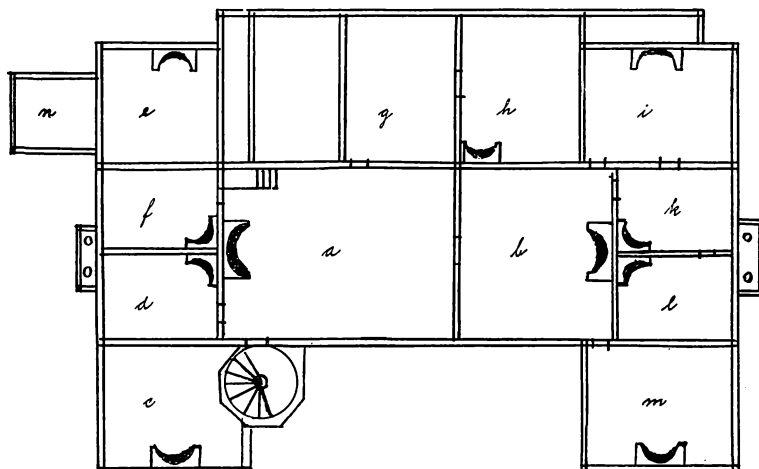
Plan af slottets 1. stokværk i 17. årh. Efter samtidig blyantstegning i landsarkivet i Åbenrå. a: forstue, b, c, e: gemakker, f: kammer, g: spisekammer, h: barne- og tyendekammer, i: køkken, k, l, m: forvalterens stuer, n: kabinet.
