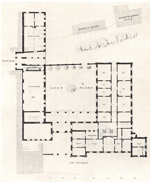
Afb. 17. Stueplan over Skolen i dens endelige Skikkelse.
