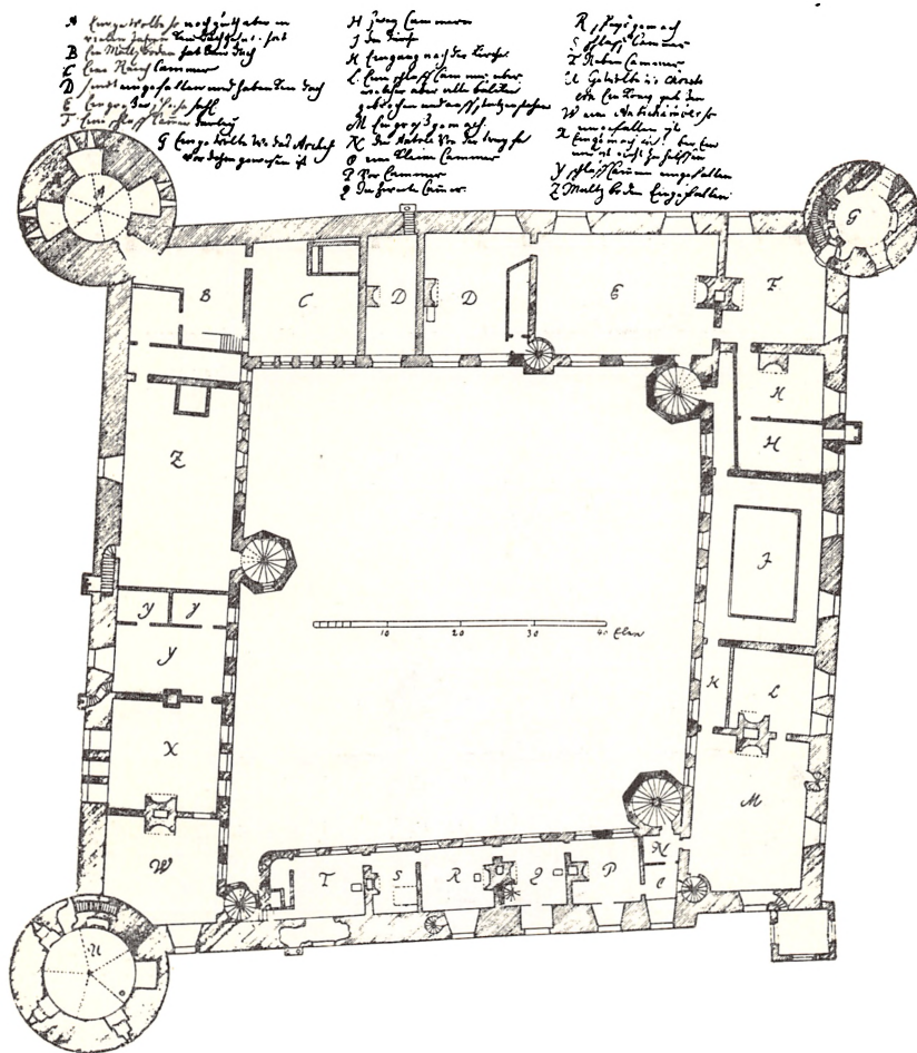
Opmaalingen fra ca. 1700 af 1. Sal. Vest opad. I Taarnet nederst til Venstre er et Plan af Christian II's Fængselsrum med Trappen op gennem Muren.
