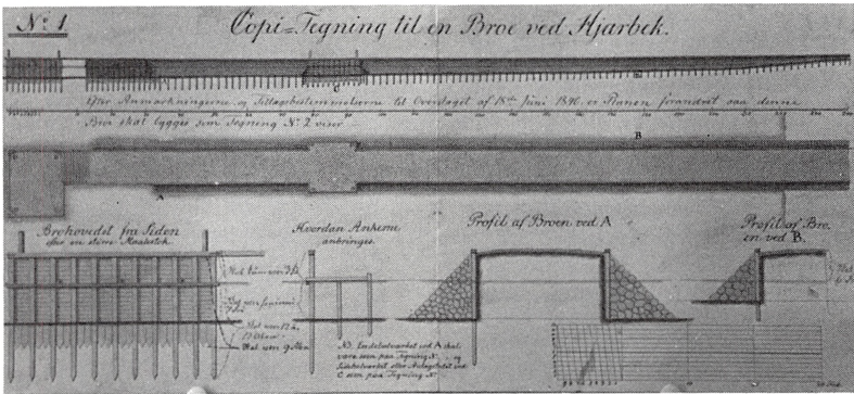
Tegninger til Hjarbæk havn fra 1840'erne. Originaler på Stadsingeniørens kontor i Viborg.
