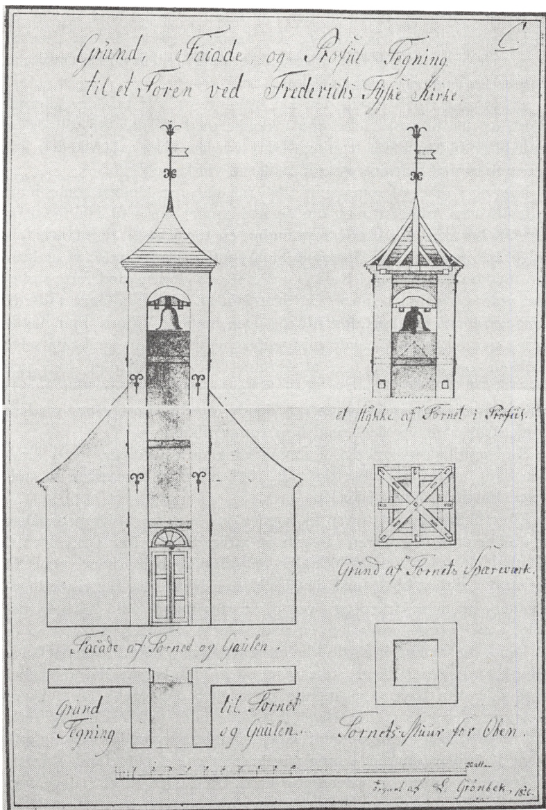
Murermester L. Grønbæks forslag til et tårn på Frederiks kirke 1826. Rigsarkivet.
