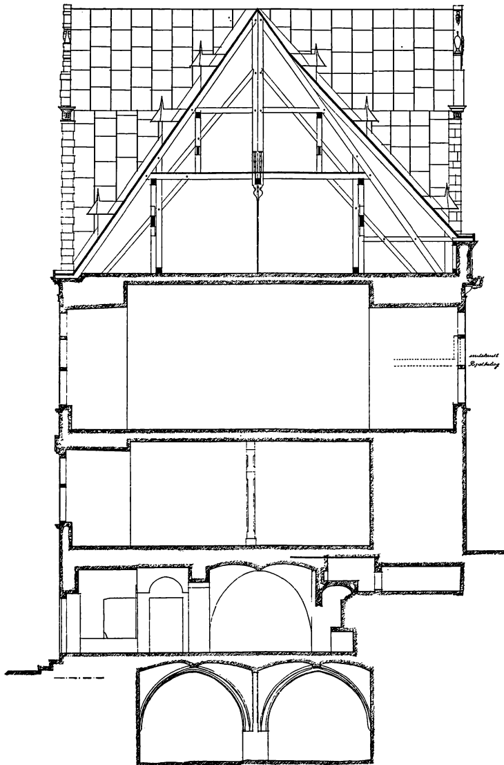
15. SNIT GENNEM VESTFLØJENS ÆLDSTE DEL MED DEN MIDDELALDERLIGE KÆLDFER. 1:1200
