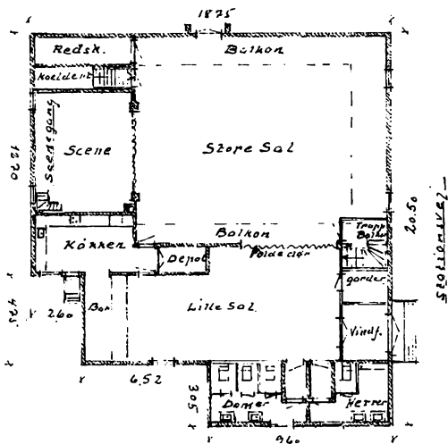
Efter Ombygningen 1970
