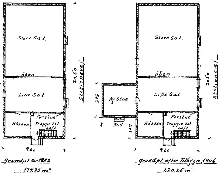
Grundtegning 1882
