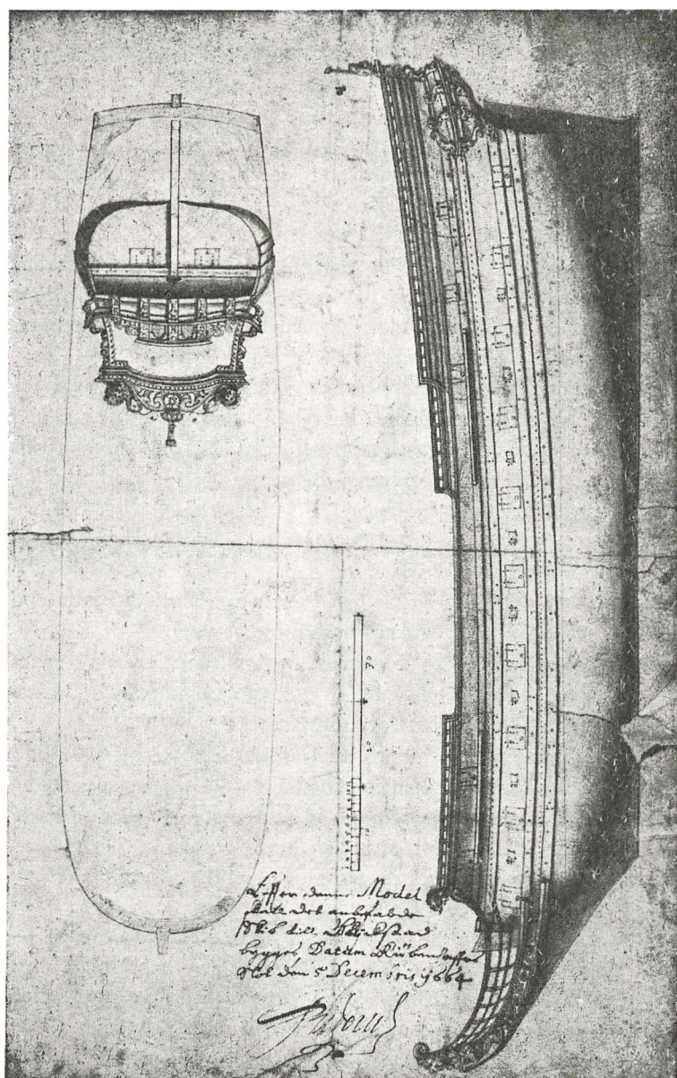
Fig. 1. Kgl. approberet tegning i Søetatens kort- og tegningsamling til dansk fregat fra 1664 (Des. A nr. 931).
