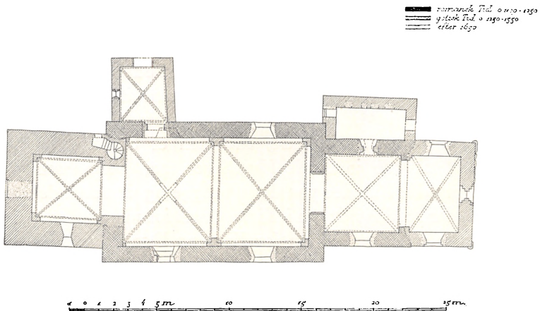
Jørlunde Kirke. Grundplan.
