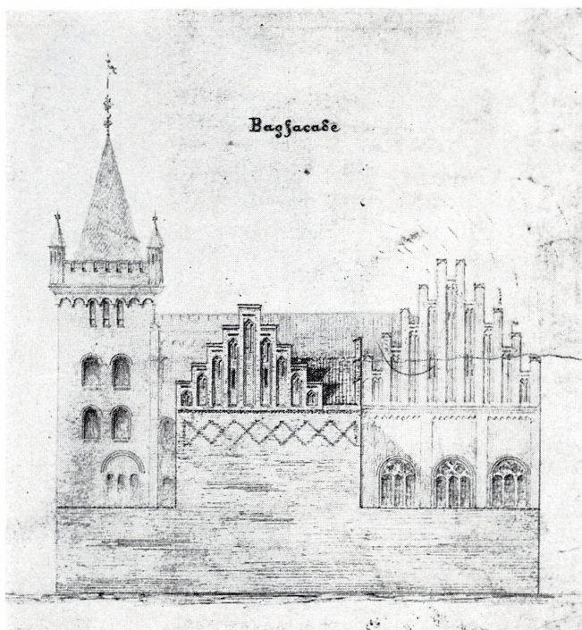
Fig. 29 b er den anden halvdel af tegningen, hvor fig. 29 a er placeret til venstre. Det viser bagfacaden. Arresthusets nordgavl og to fløjmur lukker ligesom hele komplekset af fra omverdenen. Denne gavl kan ikke ses mere, da man senere har bygget en retsbygning op ad den.
