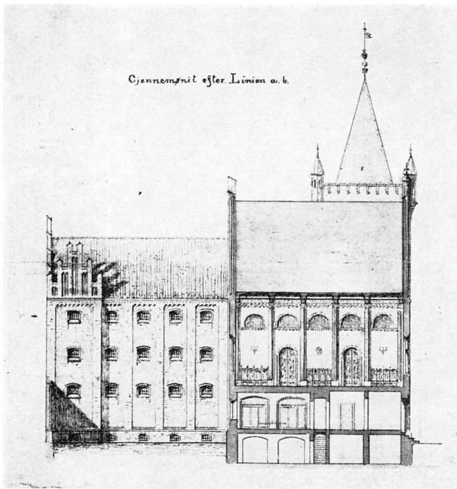
Fig. 29 a er en snittegning af byggeriet i dets endelige udformning set fra vest.
