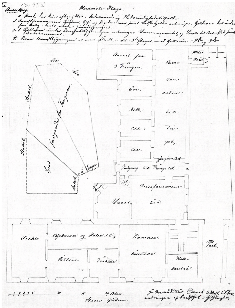
Fig. 11 og 12. Tekst til »Hr. Overauditor Crones udkast til forandring af rådhuset i Helsingør« (står nederst t. v. på begge tegninger). Øverst på I står: Underste Etage (stueplan). Anmærkning.
