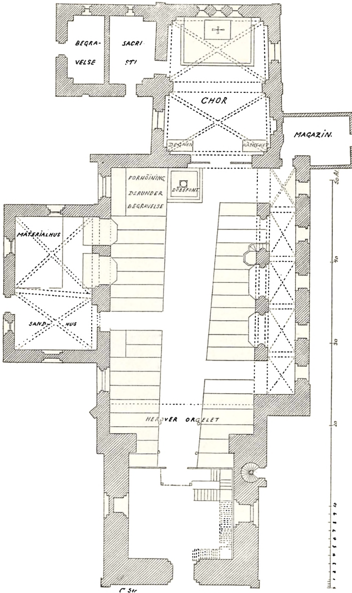
Fig. 8. Grundplan af Stubbekøbing Kirke efter Arkitekt V. Tvedes Tegning af 1861, der beror i Nationalmuseet.
