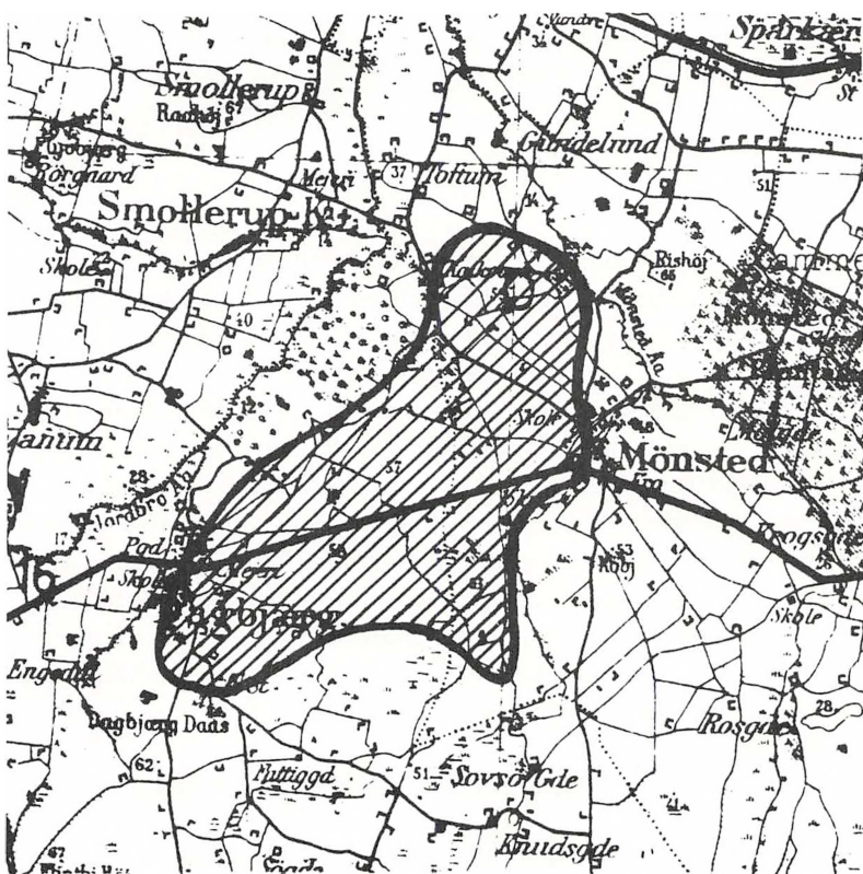
Kalkhorstens udstrækning angivet ved skravering.
