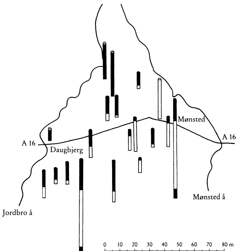
Brøndboringer i Daugbjerg-Mønsted-området. Forklaring: ses teksten. Diagrammet er udarbejdet af forfatteren på grundlag af Geologisk basiskort, Viborg, DGU 1976.
