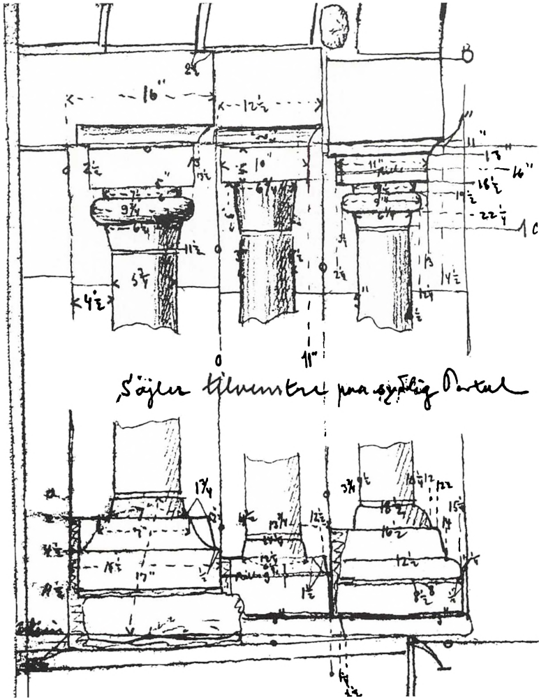
C. M. Smidts tegning og opmåling af søjleparti. Fra opholdet i Tapdrup i 1910. Nationalmuseets arkiv.
